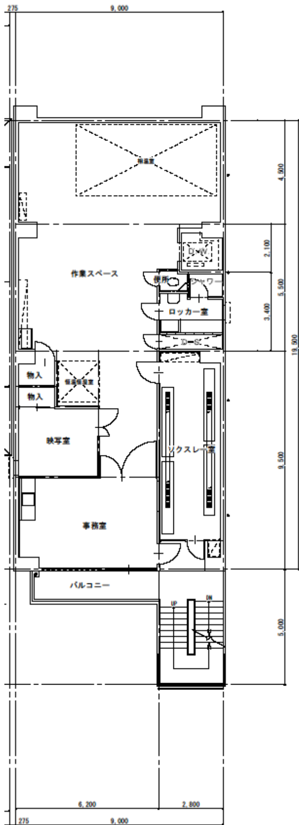
3階平面図
