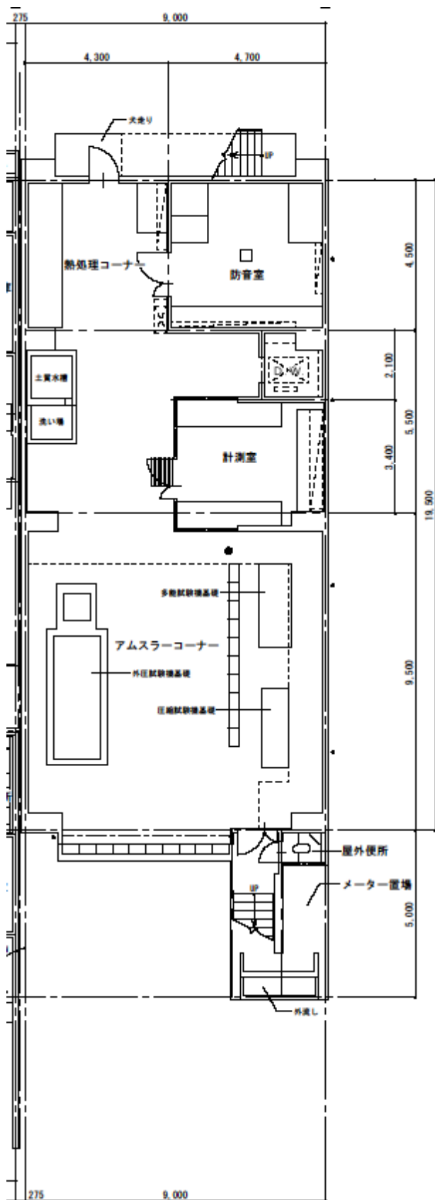
1 階平面図
