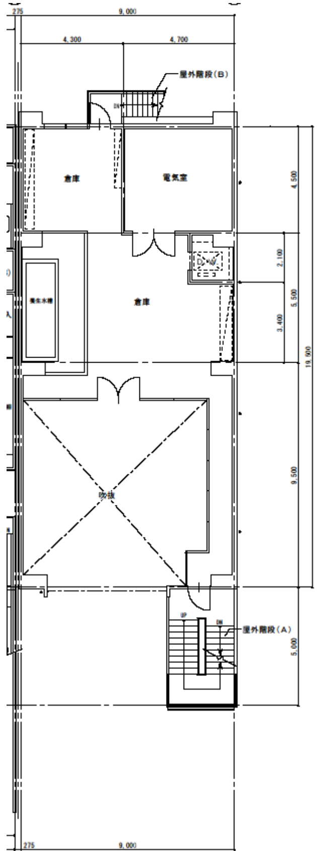
2 階平面図
